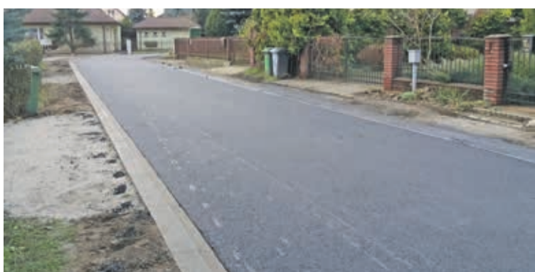
Fot. Przebudowa ul. Fiołkowej w Ligocie Pięknej
